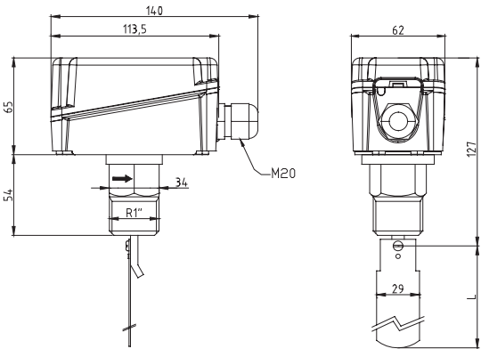
Dimensioni / Dimensions / Maßbild / Dimensions
